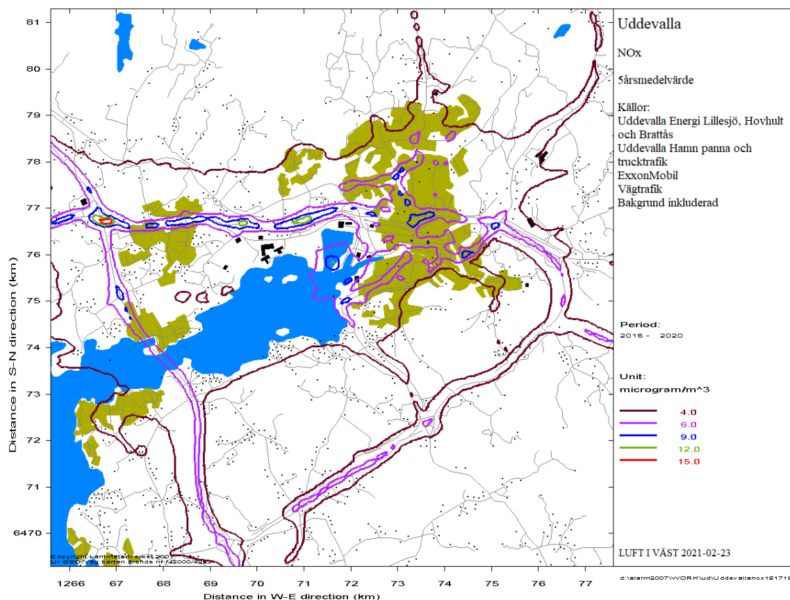
Figur F1 Resultat av en spridningsberäkning av årsmedelvärde för kväveoxider (kväveoxid + kvävedioxid) i Uddevalla baserat på data från perioden 2016–2020. Modellsystem: ALARM.
