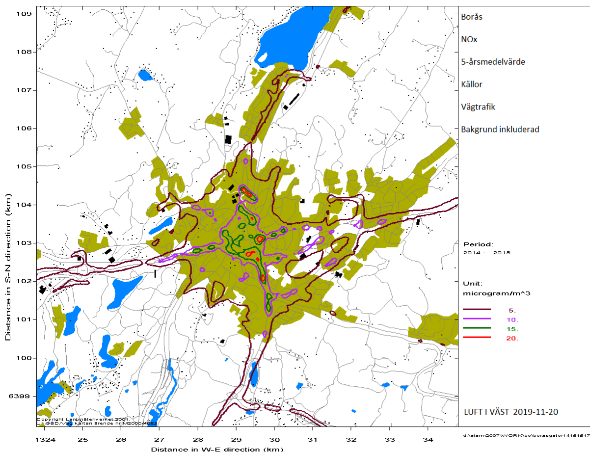
Figur B1 Resultat av en spridningsberäkning av årsmedelvärde för kväveoxider (kväveoxid + kvävedioxid) i tätorten Borås baserat på data från perioden 2014–2018. Modellsystem: ALARM.
